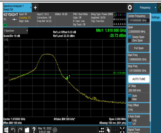
Band2-5MHz-QPSK-19175-1RB#24
