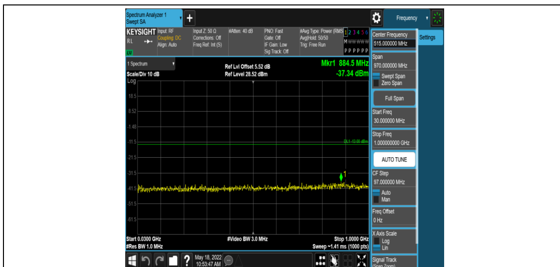
Band2-20MHz-QPSK-18900-1RB#0-Range3:30~1000MHz
