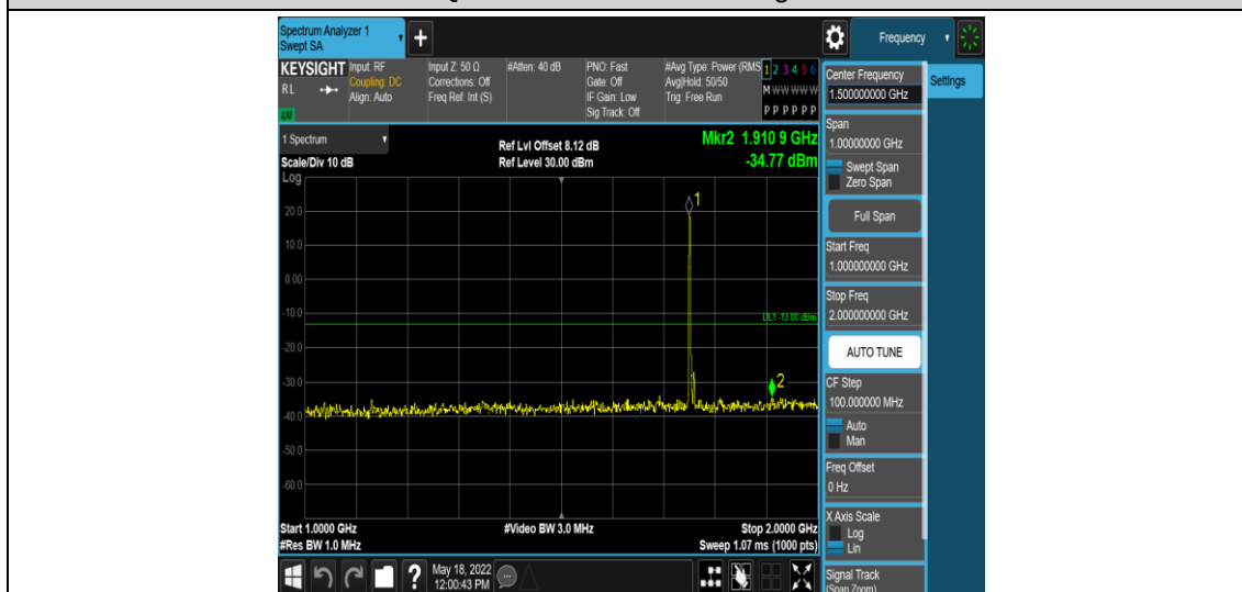
Band4-5MHz-QPSK-20375-1RB#0-Range4:1000~2000MHz
