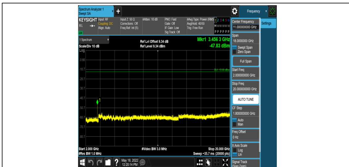
Band4-10MHz-QPSK-20175-1RB#0-Range5:2000~20000MHz
