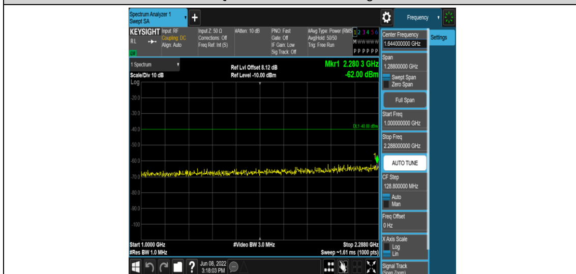
Band40-5MHz-16QAM-39200-1RB#0-Range4:1000~2288MHz
