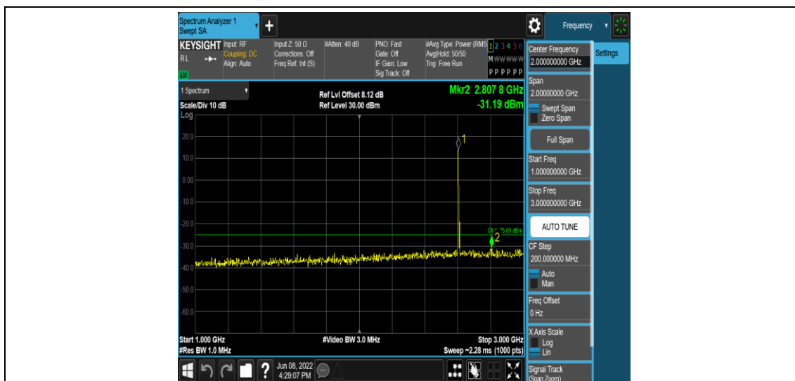
Band41-5MHz-QPSK-40740-1RB#0-Range4:1000~3000MHz
