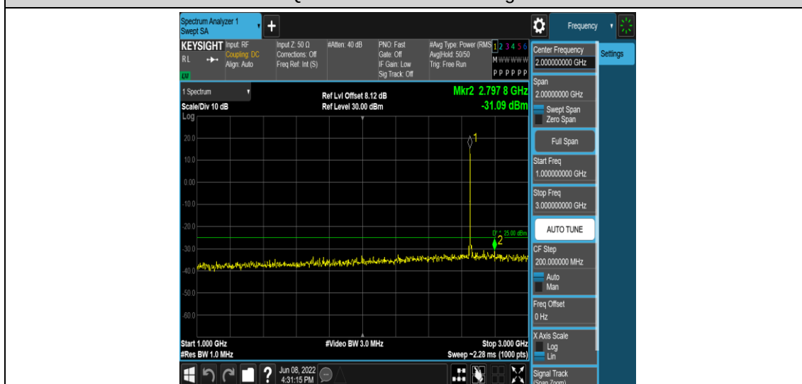
Band41-5MHz-QPSK-41215-1RB#0-Range4:1000~3000MHz
