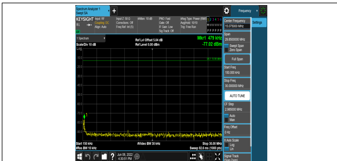
Band41-5MHz-QPSK-41215-1RB#0-Range2:0.15~30MHz
