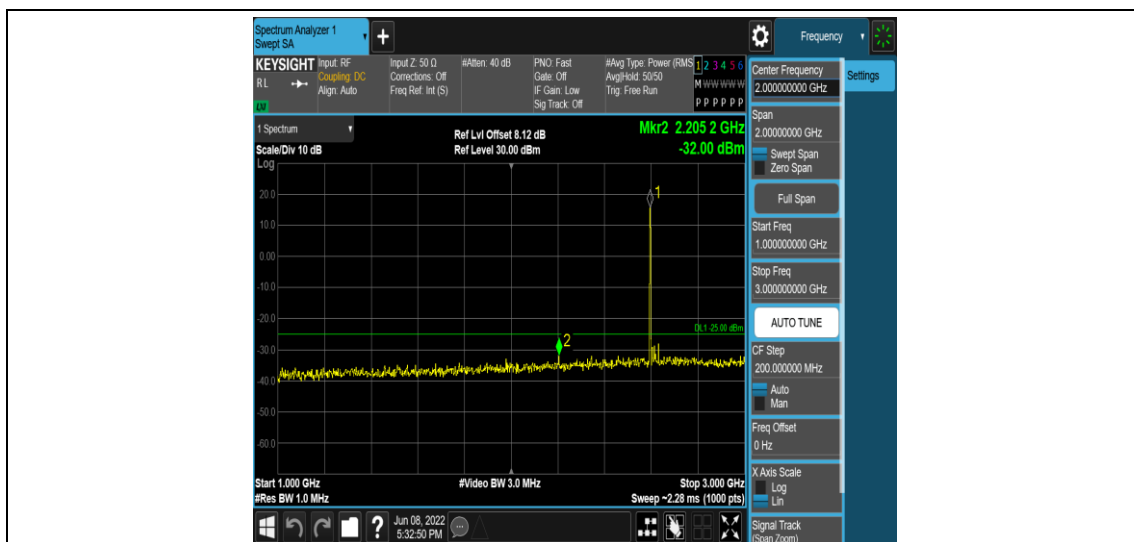
Band41-20MHz-QPSK-40740-1RB#0-Range4:1000~3000MHz
