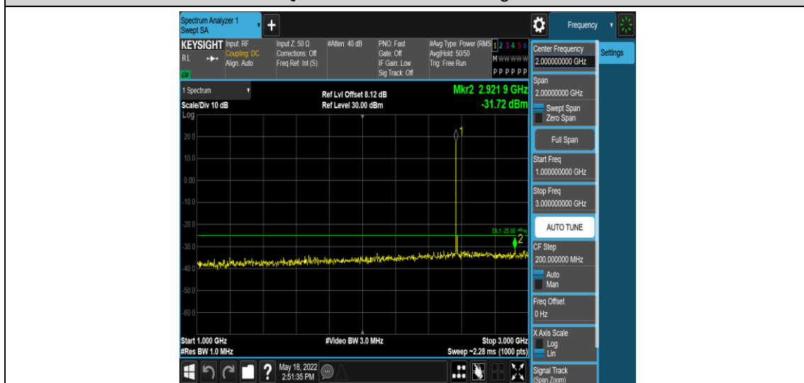
Band7-5MHz-QPSK-21425-1RB#0-Range4:1000~3000MHz
