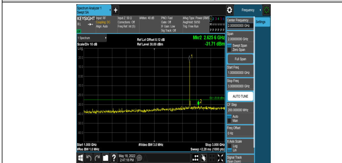
Band7-5MHz-QPSK-20775-1RB#0-Range4:1000~3000MHz
