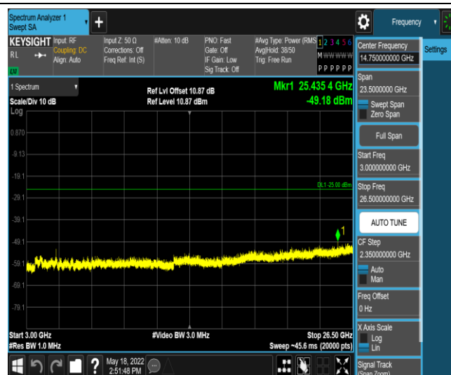
Band7-5MHz-QPSK-21425-1RB#0-Range5:3000~26500MHz
