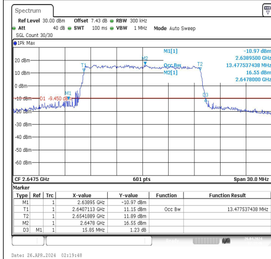
41(2555-2655)-15MHz-QPSK-41165-75RB#0-PA SS
