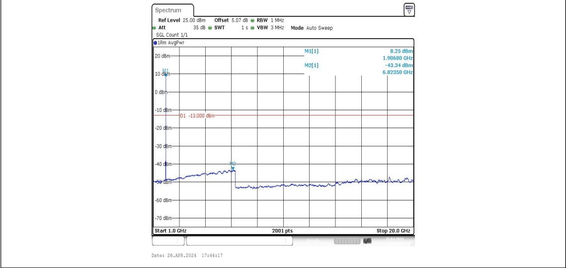
Band2-9538-1-1000~20000MHz-PASS
