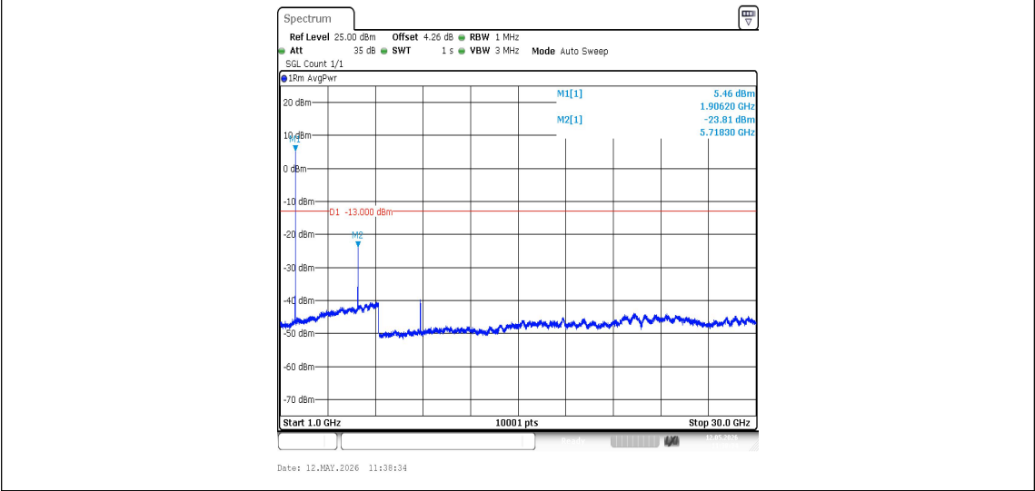
Band2-9538-3-1000~30000MHz-PASS
