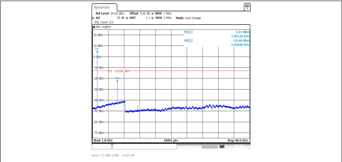
Band2-9262-1-1000~30000MHz-PASS
