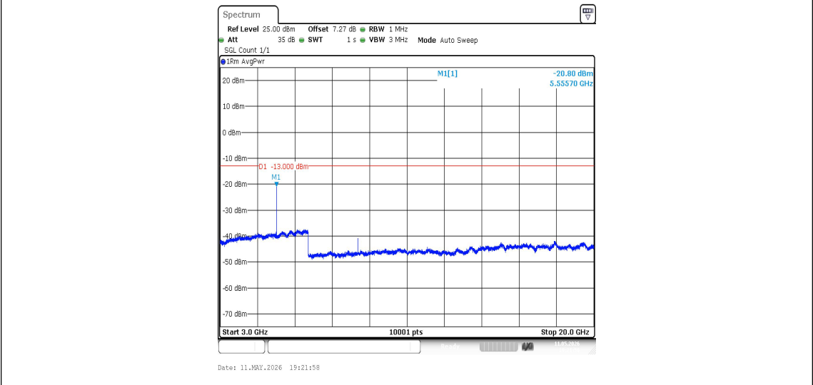
Band2-9262-1-3000~20000MHz-PASS
