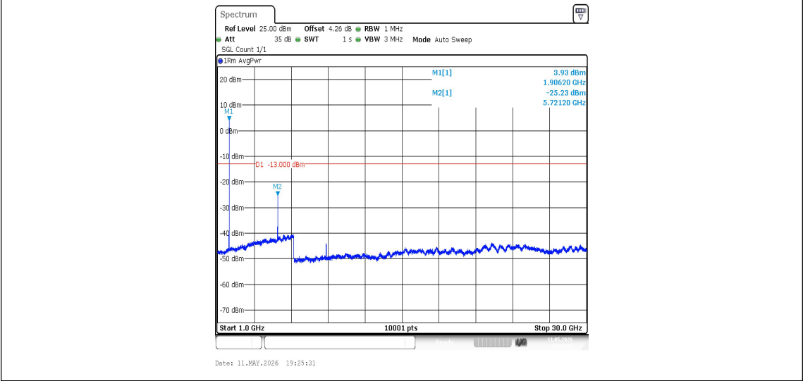
Band2-9538-1-1000~30000MHz-PASS
