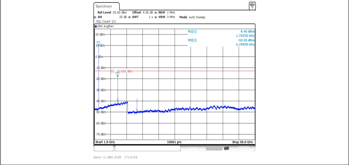
Band4-1413-1000~30000MHz-PASS
