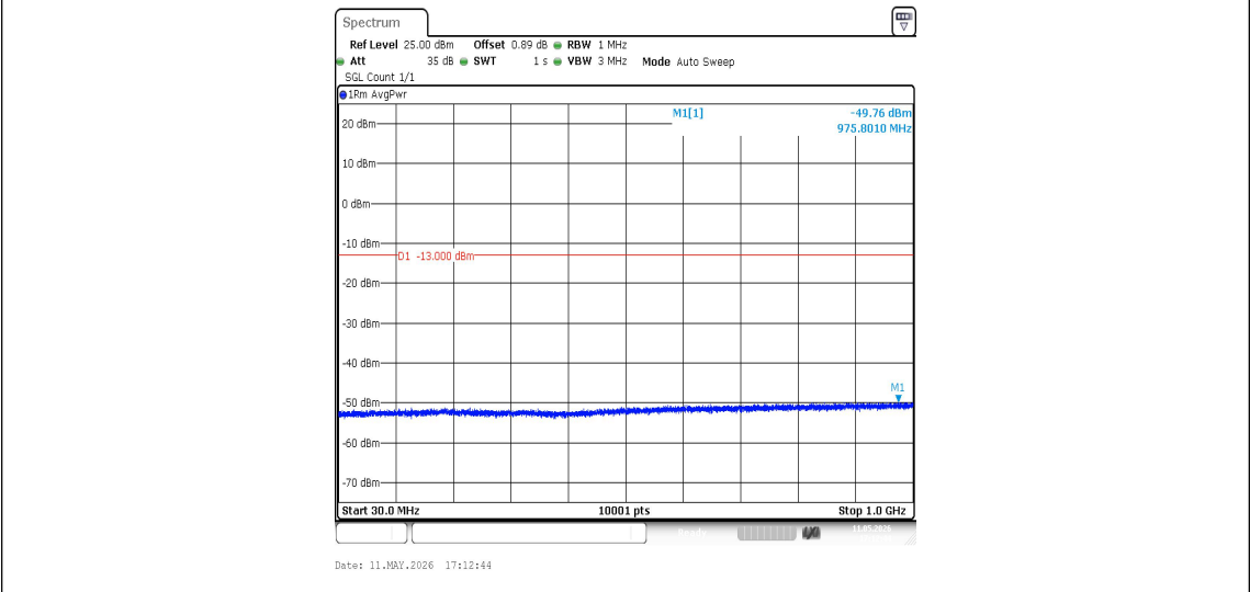
Band4-1413-30~1000MHz-PASS
