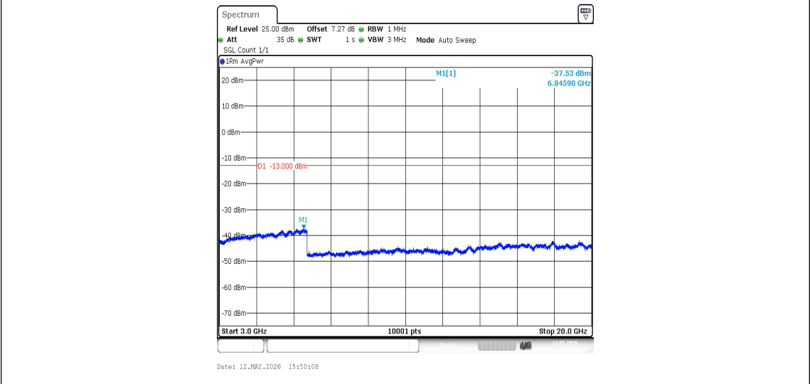
Band4-1413-3-3000~20000MHz-PASS
