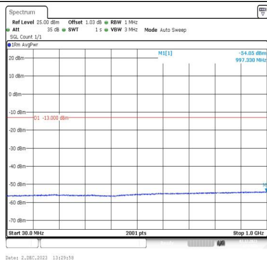
Band2-9400-1-30~1000MHz-PASS
