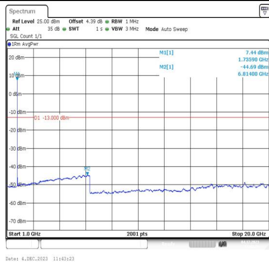
Band4-1413-4-1000~20000MHz-PASS
