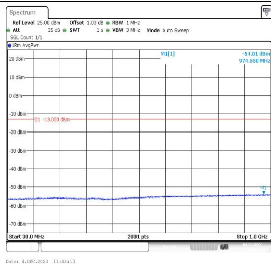
Band4-1413-4-30~1000MHz-PASS
