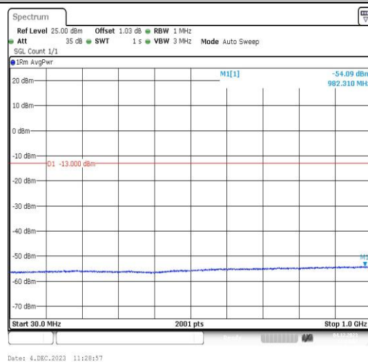
Band4-1312-1-30~1000MHz-PASS
