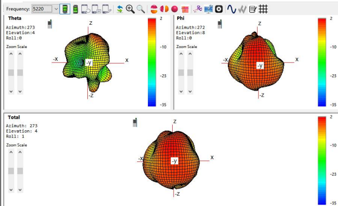
5G WIFI: 5220Mhz
