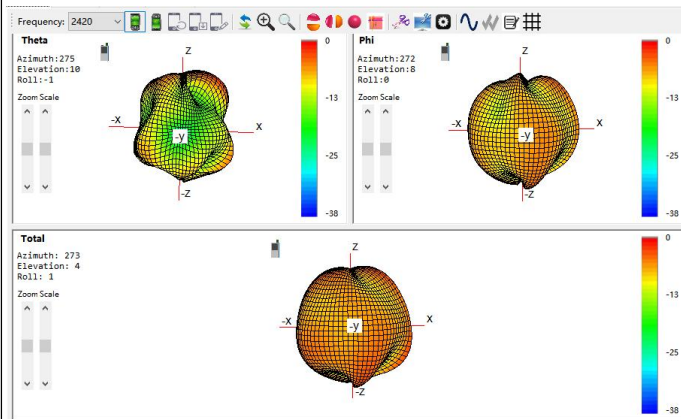
2.4G WIFI/BT: 2420Mhz
