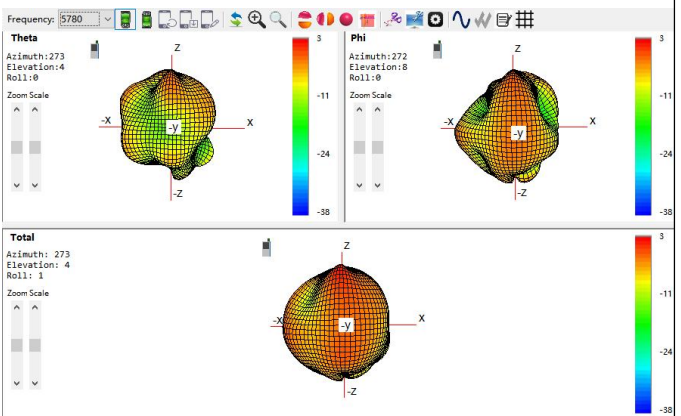
5G WIFI: 5780Mhz
