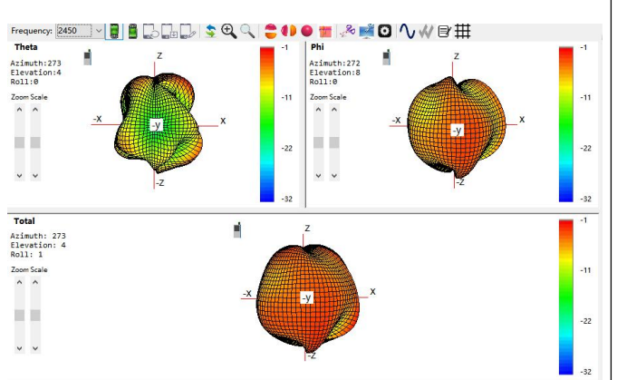
2.4G WIFI/BT: 2450Mhz
