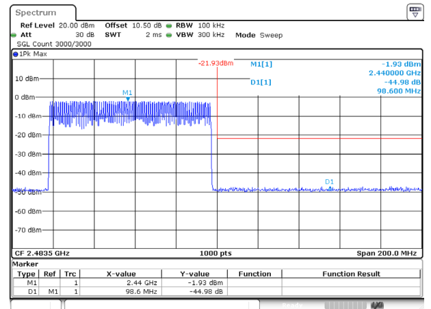
DH1_Hopping_Upper
