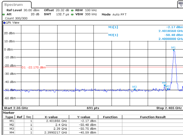
DH1_Ant1_Low_2402
