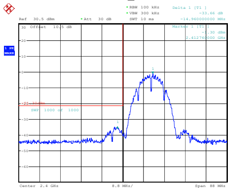
802.11b_2412MHz
