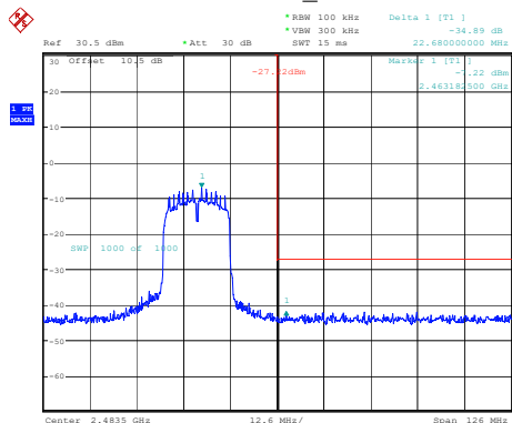
802.11n20_2462MHz
