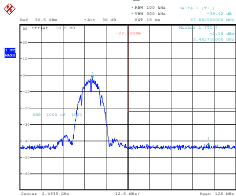
802.11b_2462MHz
