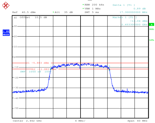
802.11n20_2462MHz
