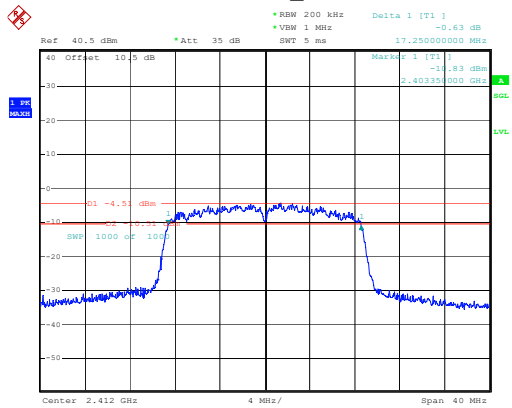
802.11n20_2412MHz
