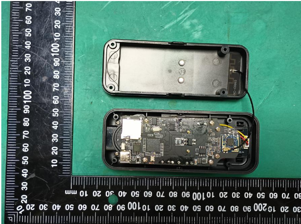
Wi-Fi ANT
