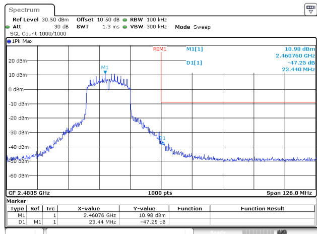
802.11n20_2462MHz
