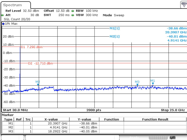
802.11b_2462MHz
