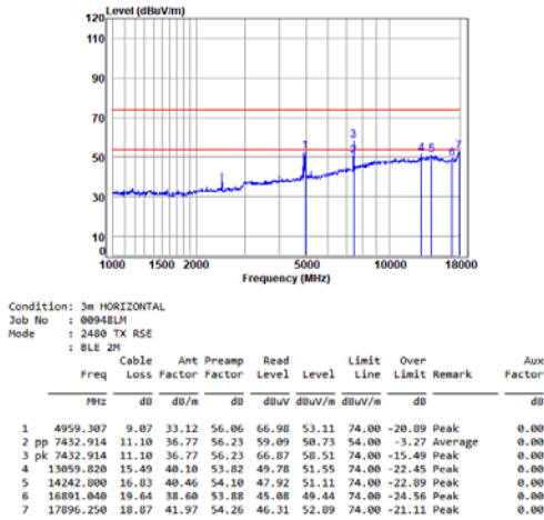
BLE_2M_TX_CH_39_Horizontal
