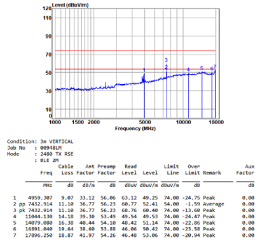
BLE_2M_TX_CH_39_Vertical
