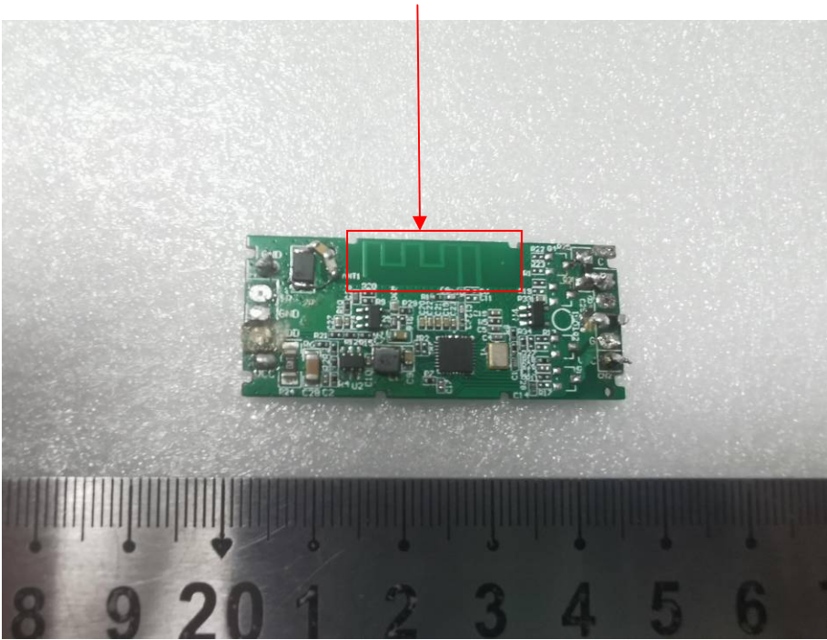
Antenna
