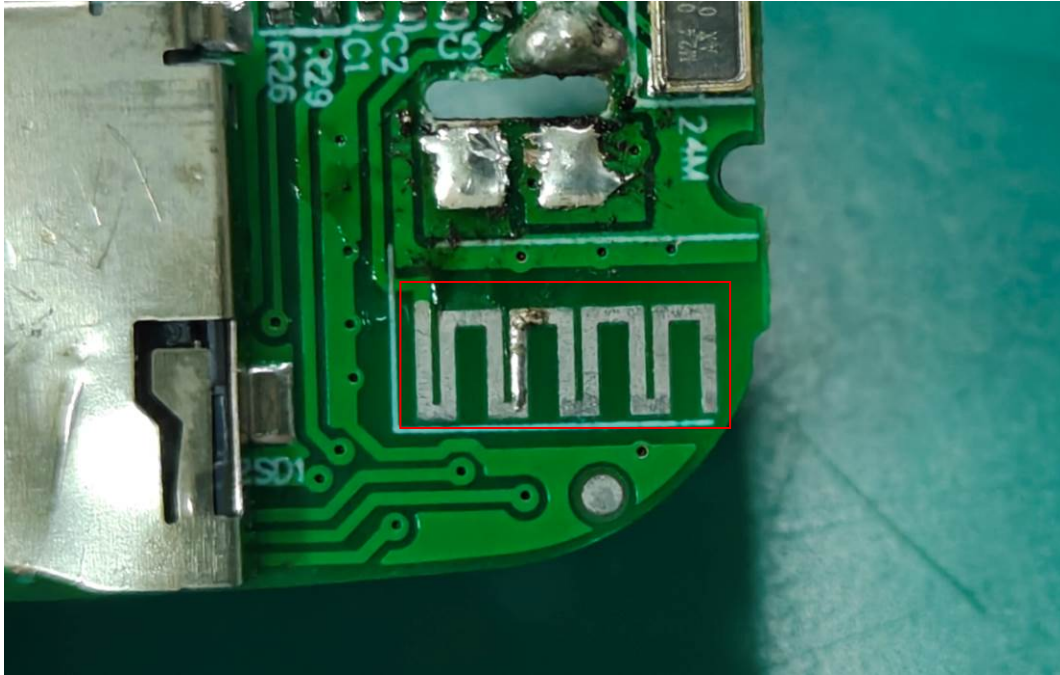
BT ANT
