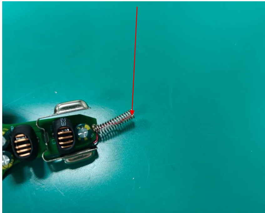
FM ANT
