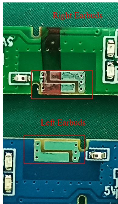
Antenna
