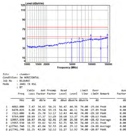
BT_DH5_TX_CH_39_Horizontal
