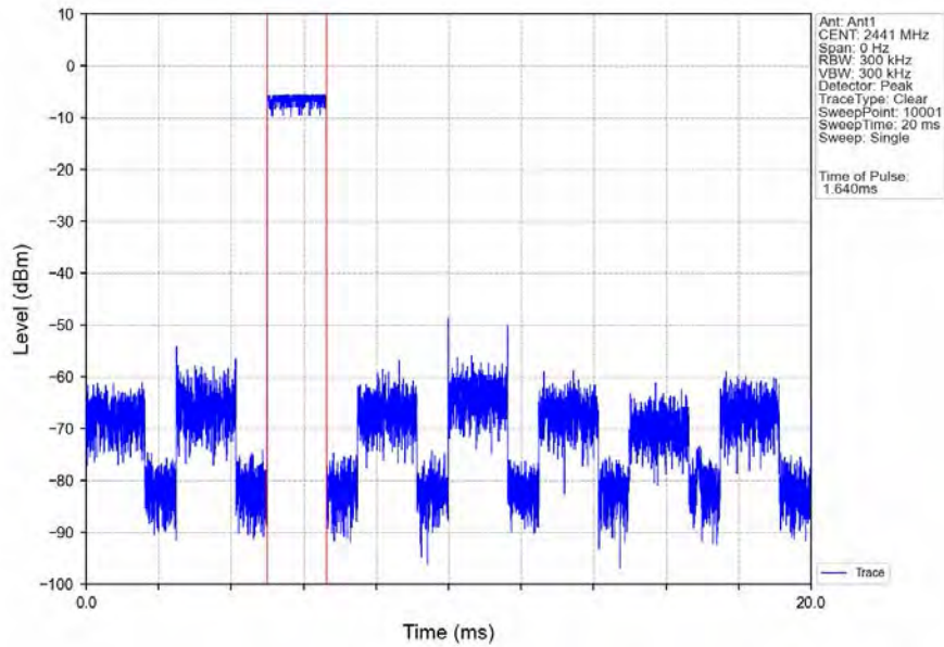
GFSK_DH3_HOPP_Ant1_NTNV
