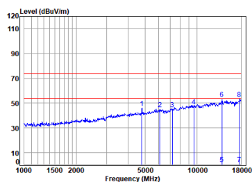
2.4G SRD_TX_CH_L_Horizontal
