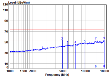
2.4G SRD_TX_CH_H_Horizontal
