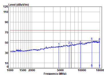
2.4G SRD_TX_CH_L_Vertical
