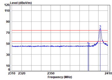
2.4G SRD_TX_CH_L_Vertical
