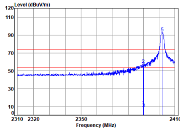
2.4G SRD_TX_CH_L_Horizontal
