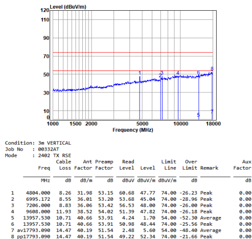
2.4G SRD_TX_CH_L_Vertical
