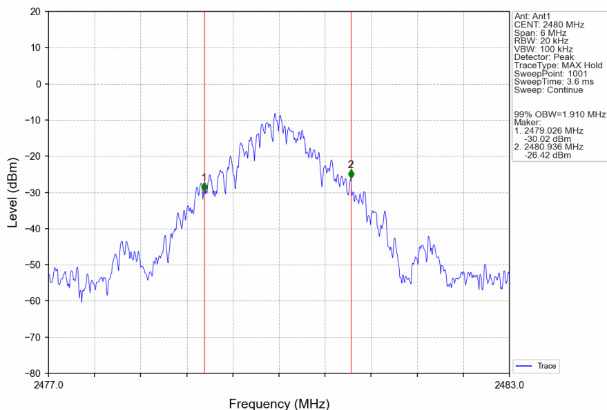
TX_HCH_2480MHz_Ant1_NTNV
