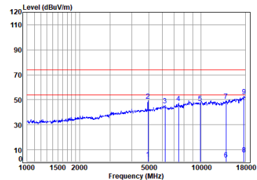
2.4G SRD_TX_CH_H_Vertical
