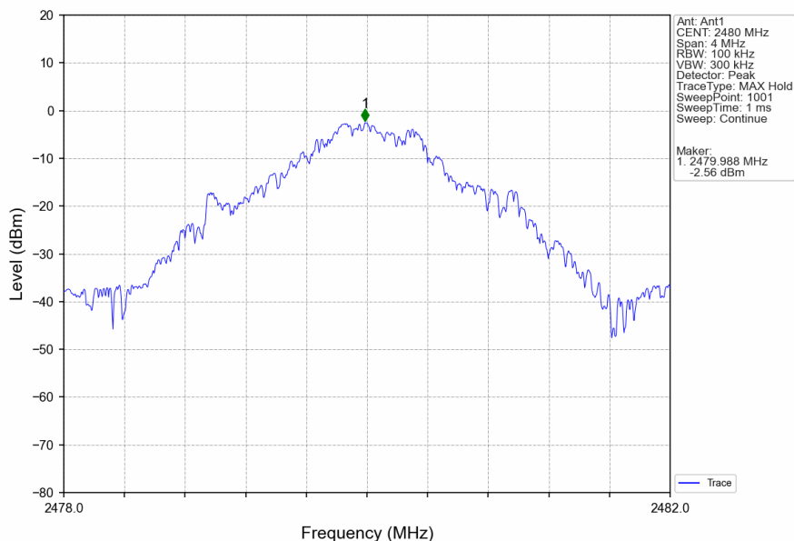
TX_HCH_2480MHz_Ant1_NTNV
