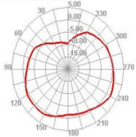
2440.000MHz H
