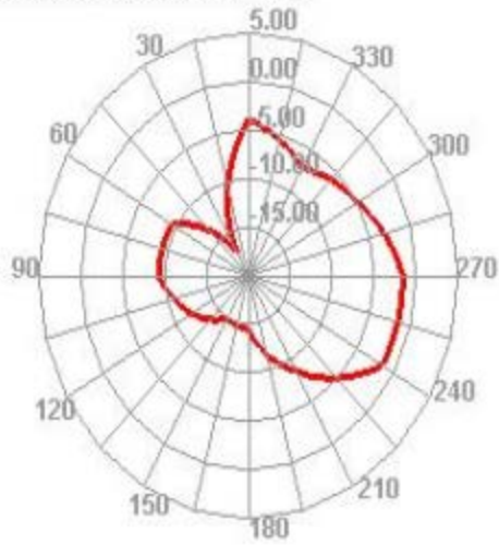
2430.000MHz E1
