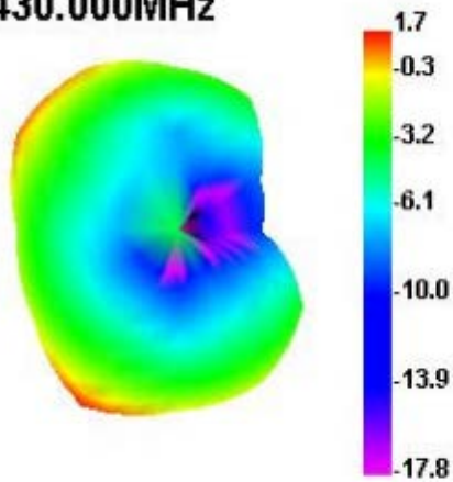
2430.000MHz
