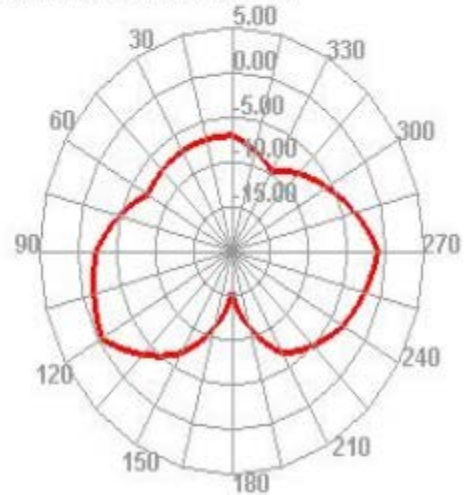
2420.000MHz E2
