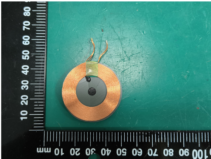
WPT ANT
