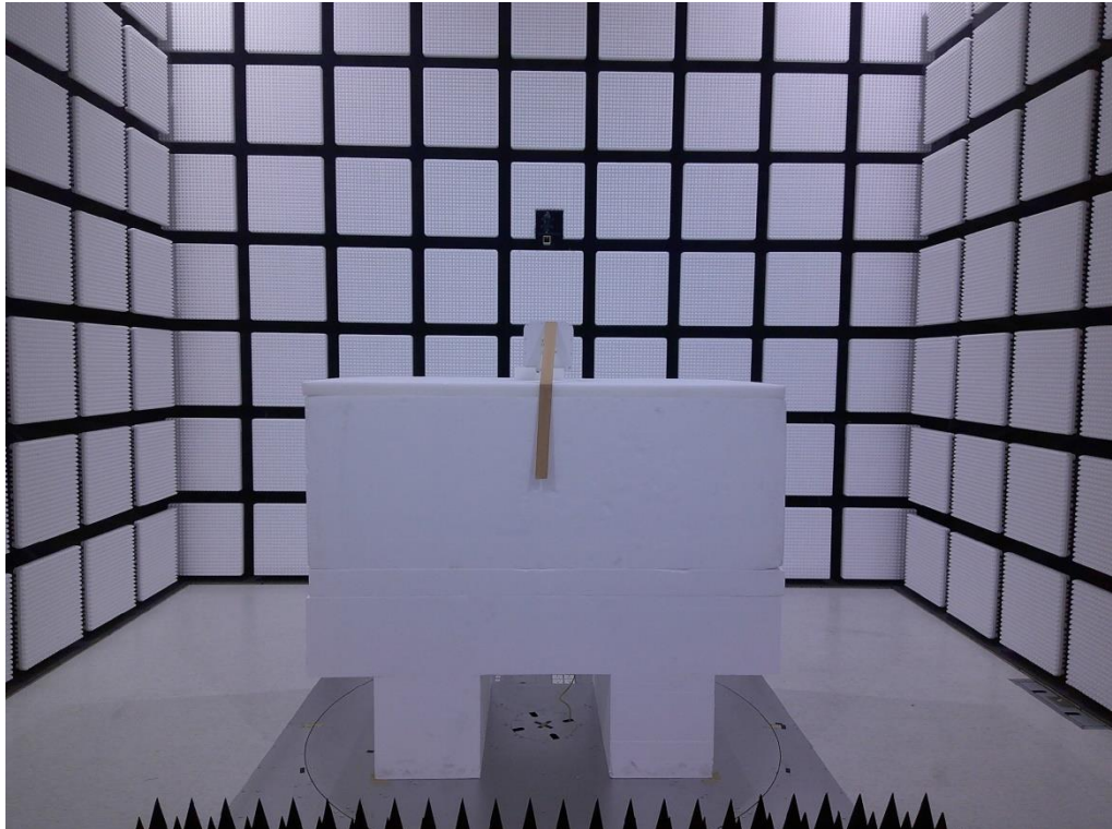
Radio 2 (1TX)
