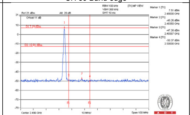
CH 39 Band edge
