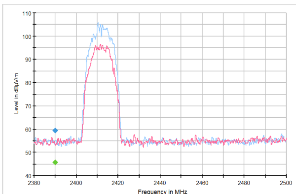
Figure 3. Band Edge
