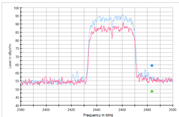
Figure 10. Band Edge
