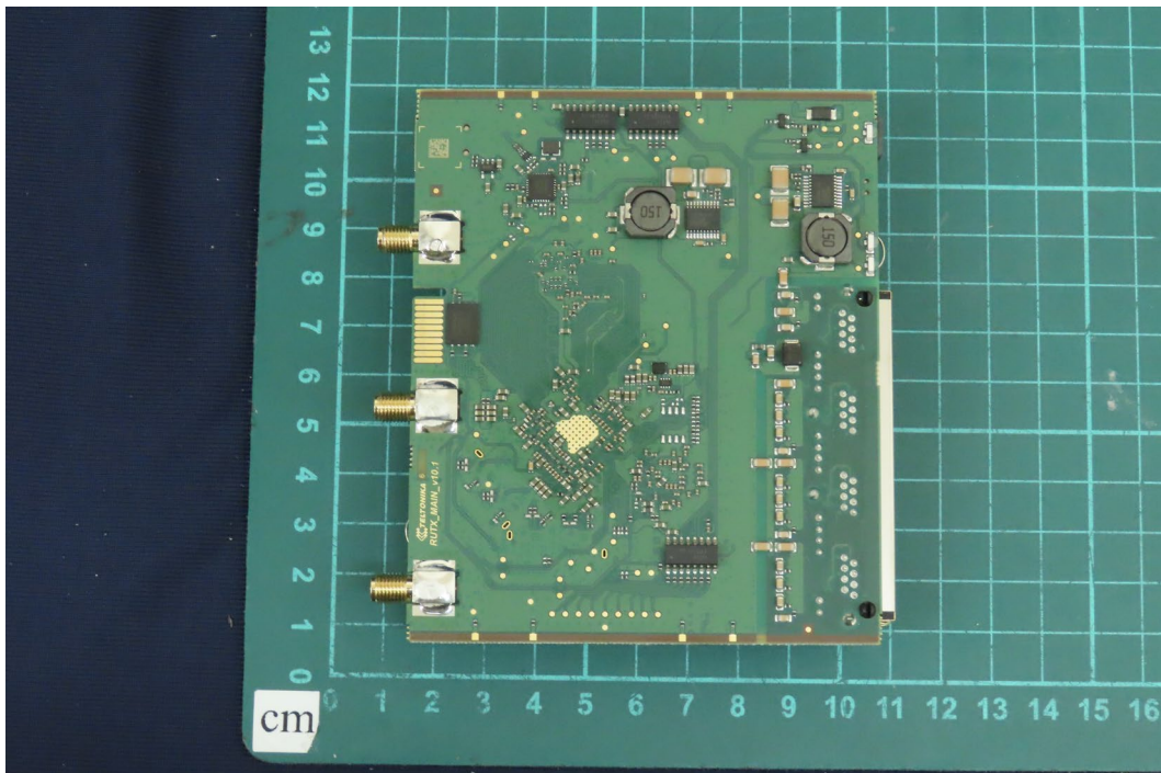
(30) EUT Photo
