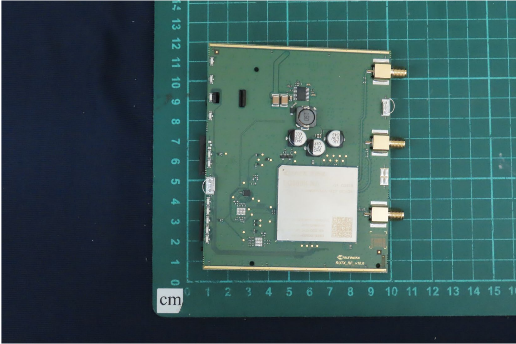
(24) EUT Photo
