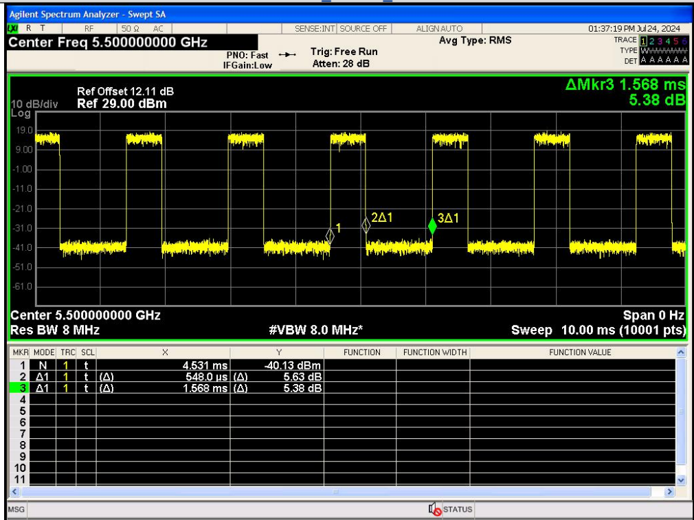
IEEE 802.11n_20MHz_Channel 100
