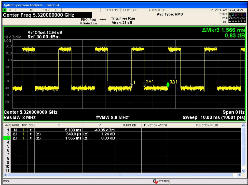
IEEE 802.11n_20MHz_Channel 64
