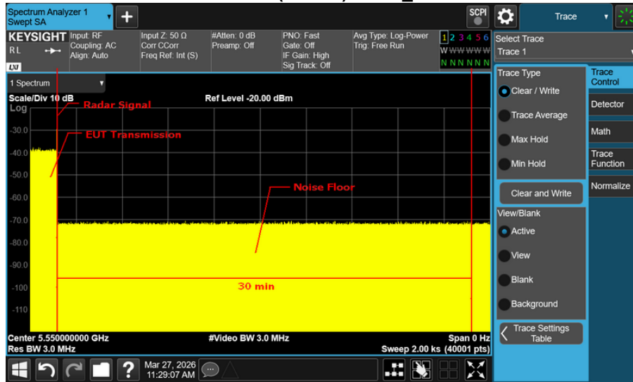
IEEE 802.11ac(VHT40) Mode_5550MHz
