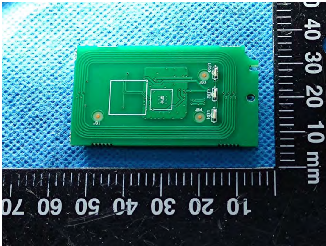
NFC Antenna
