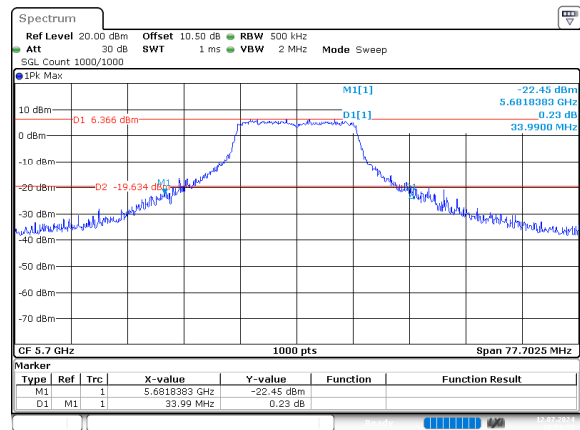
a_5700MHz_Chain 0
