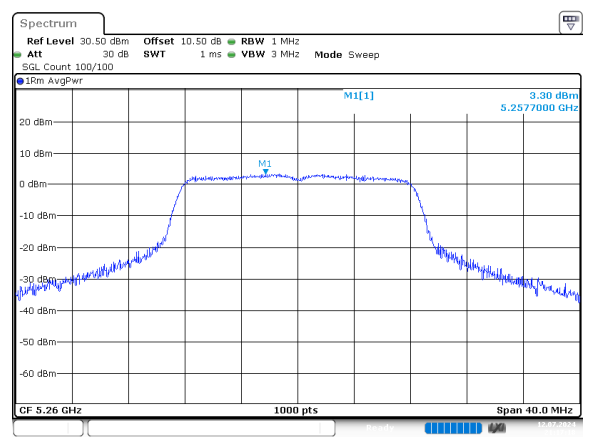
a_5260MHz_Chain 0
