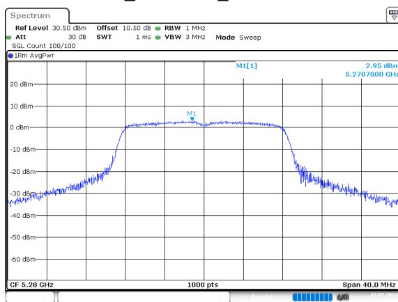
a_5280MHz_Chain 0
