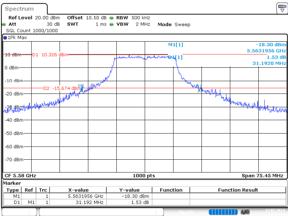
a_5580MHz_Chain 0
