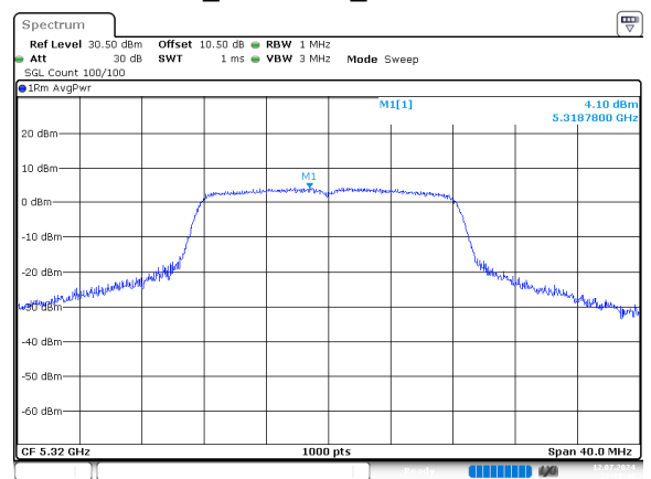
a_5320MHz_Chain 0
