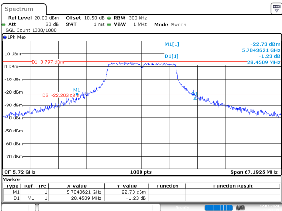
a_5720MHz_Chain 0
