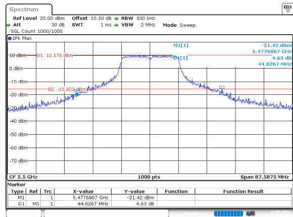
n20_5500MHz_Chain 0
