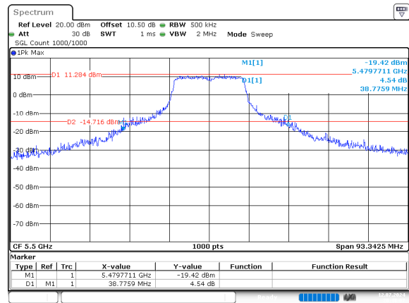
a_5500MHz_Chain 0
