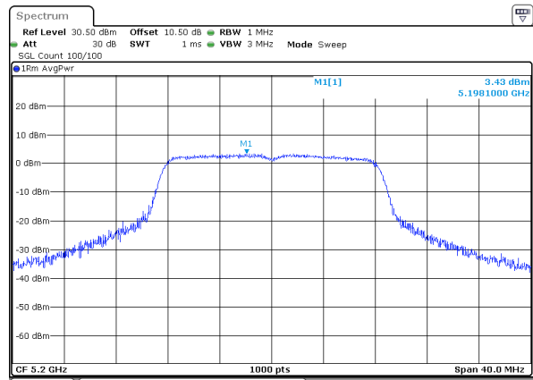
a_5200MHz_Chain 0
