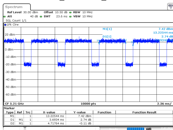
ac80_5210MHz_Chain 0
