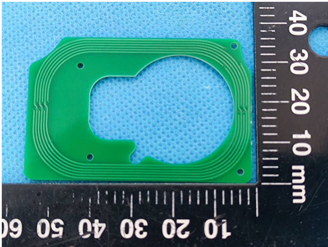
NFC Antenna-13.56M
