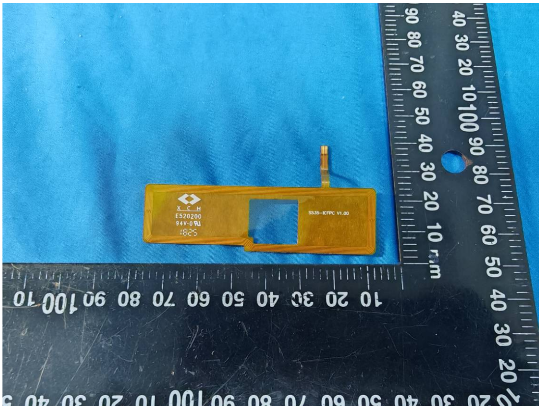
NFC Antenna(13.56MHz)
