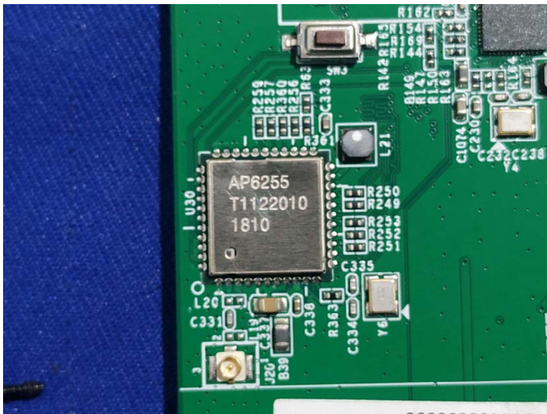
BT&WIFI Module
