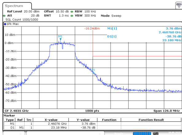
802.11n20_2462MHz
