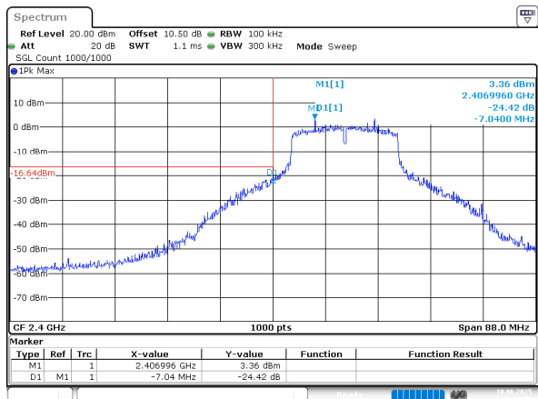
802.11n20_2412MHz
