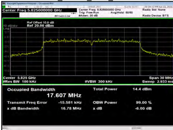
802.11n 20MHz Main 5825MHz
