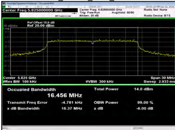
802.11a 20MHz Main 5825MHz
