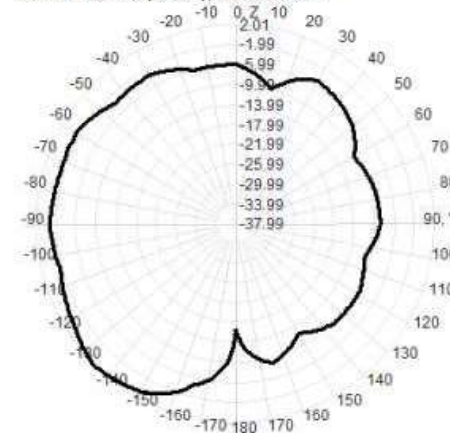
2450.0MHz Total(E2-YZ), Max=2.01dBi
