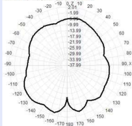
2450.0MHz Total(E1-XZ), Max=-4.11dBi
