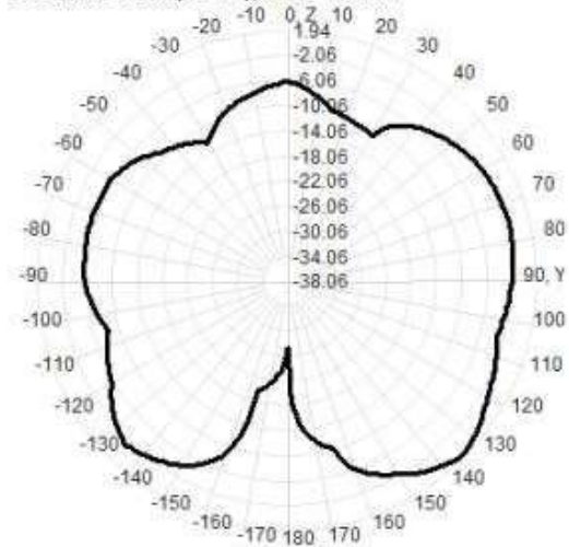
2400.0MHz Total(E2-YZ), Max= 1.32dBi
