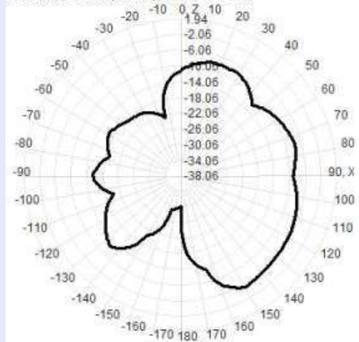
2400.0MHz Total(E1-XZ), Max=-5.35dBi
