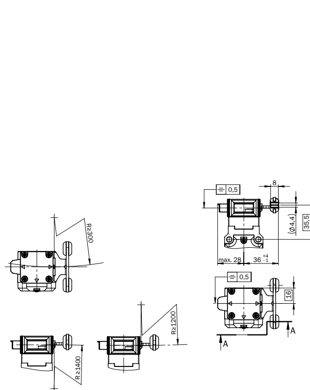
Figure 50: Min. door radii for TR110-XABT angled actuator (mm)
