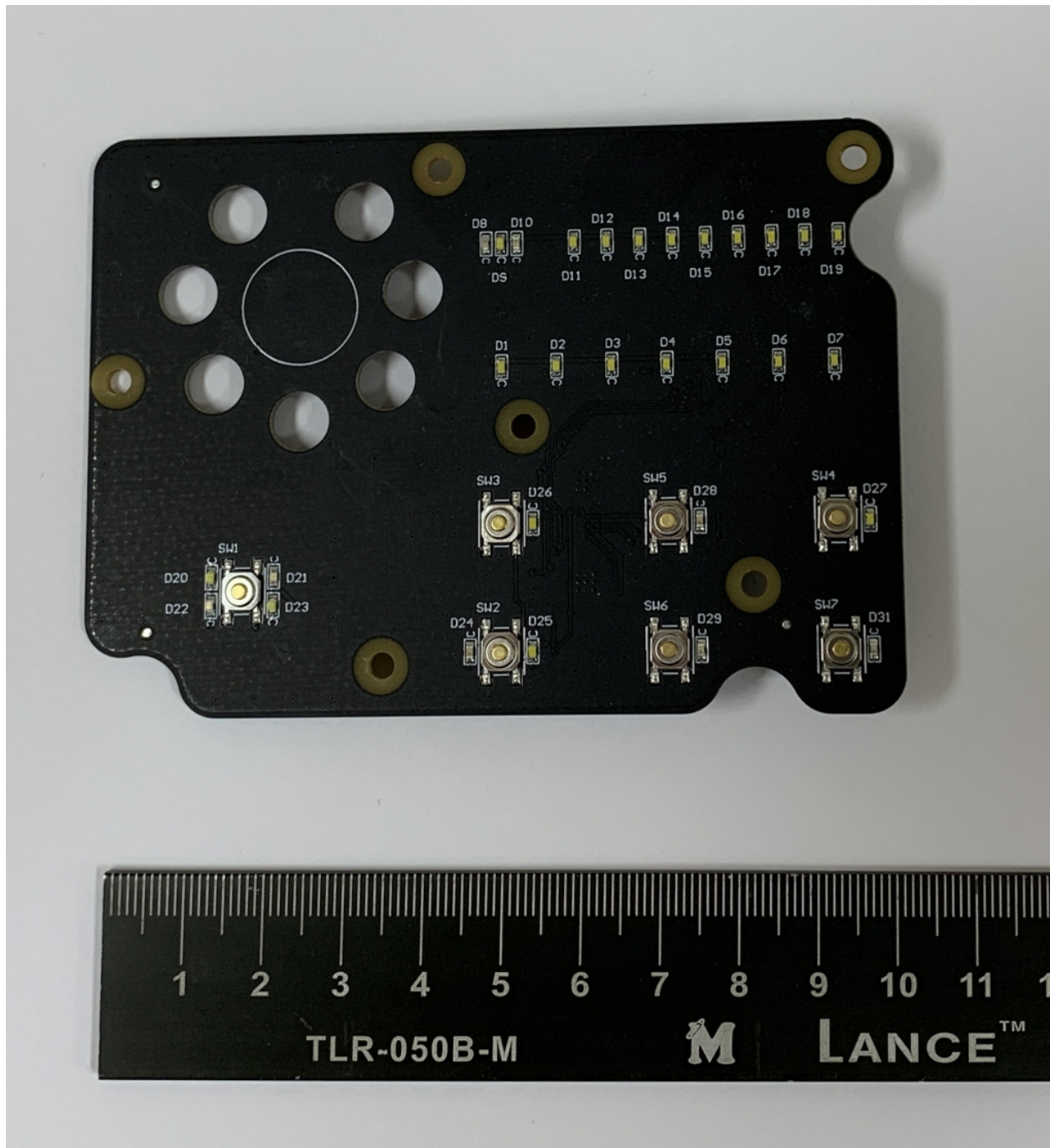
Keypad Top
