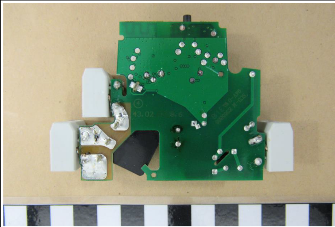
EUT INTERNAL VIEW (D)
