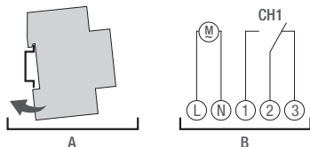
4. ábra: DIN-sínre történő felszerelés és kapcsolási rajz
