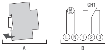
Fig. 4: Montering på DIN-skinne og koblingsskjema
