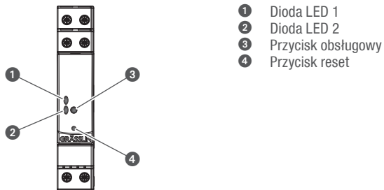
Rys. 2: Elementy wskaźnikowe i obsługowe
