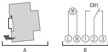
Fig. 4: Montering på DIN-skinne og koblingsdiagram
