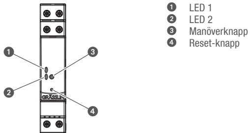
Bild 2: Indikerings- och manöverelement
