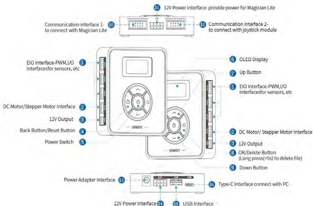
图 4.1 Magic Box 接口
