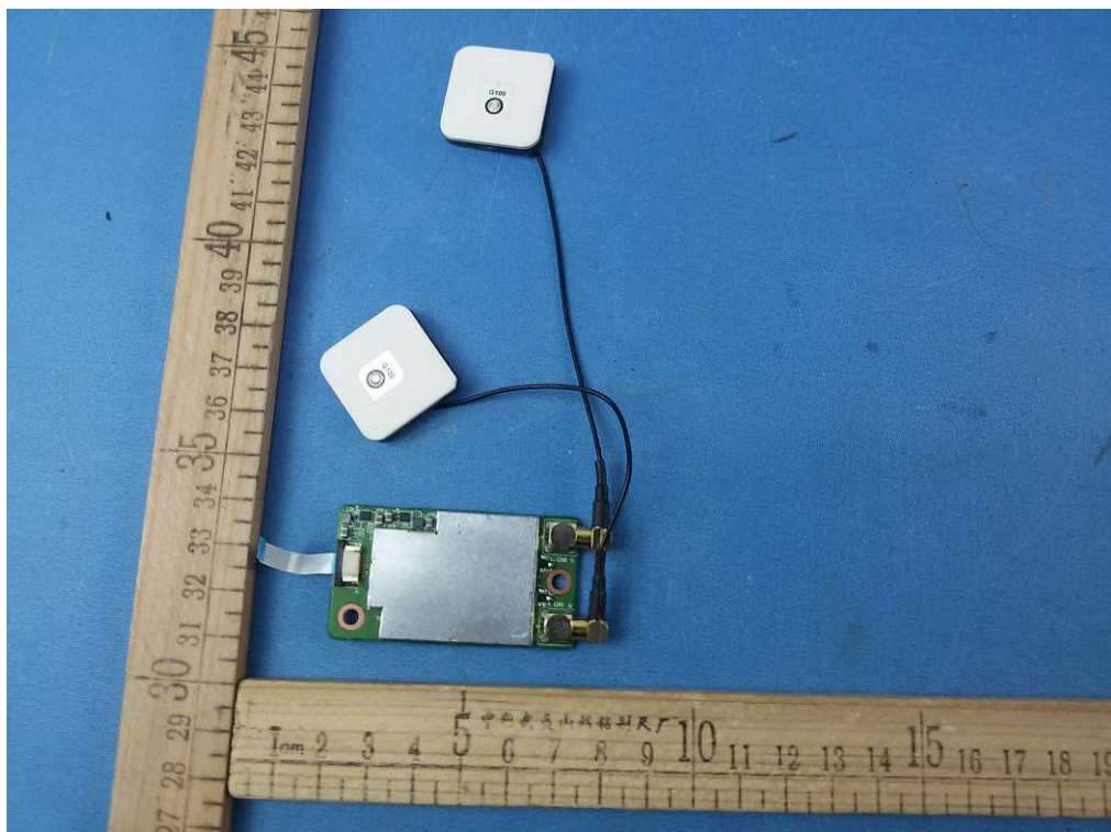
Photo 7 RX Module
