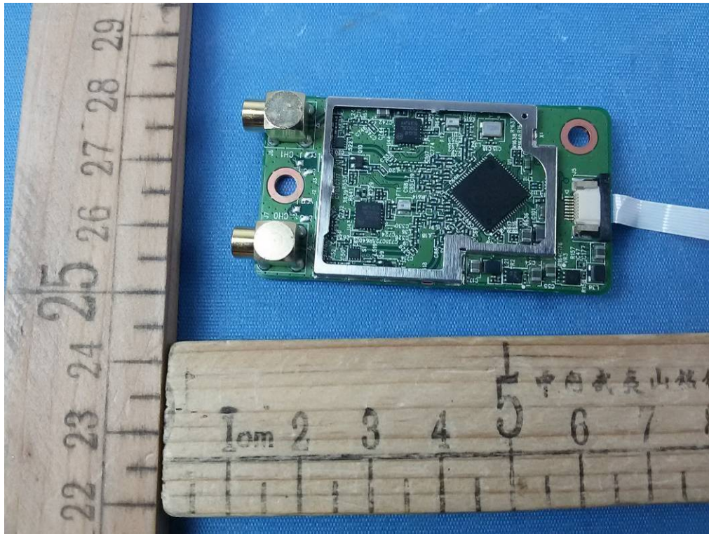
Photo 8 RX Module
